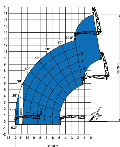
Sur stabilisateurs avec fléchette 4m (hydraulique/mécanique)
