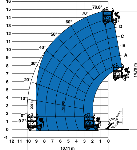
Sur stabilisateurs avec nacelle 3P-700REM 4400
